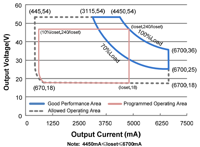
EUD-240S670DTA
