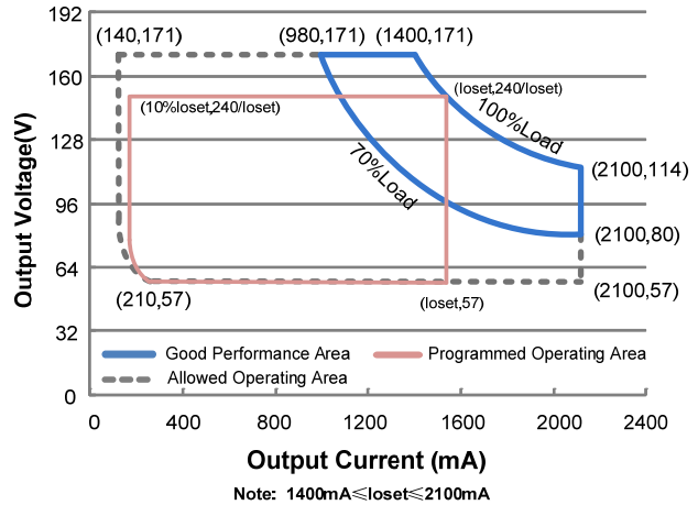
EUD-240S210DTA
